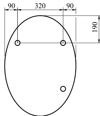
вертикальное расположение зеркала
